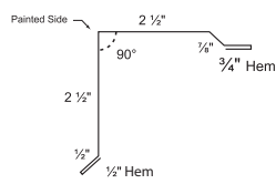
2. Mini Gable
