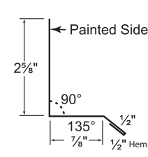
16. 4 1/2" Drip Cap
