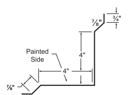
17. Eave Trim
