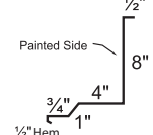
21. Side Chimney
