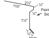
8. Drip Edge
