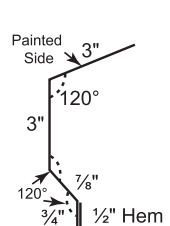
17. Eave Trim
