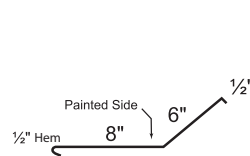
20. Bottom Chimney
