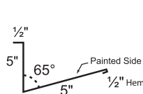
19. Top Chimney
