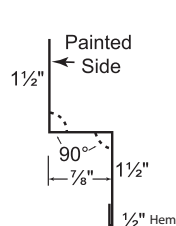
15. Double Angle
