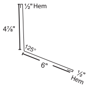
10A. Endwall
